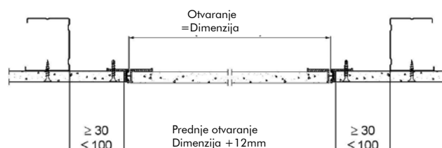
Shematski prikaz: revizijska vrata za vlažne prostorije
